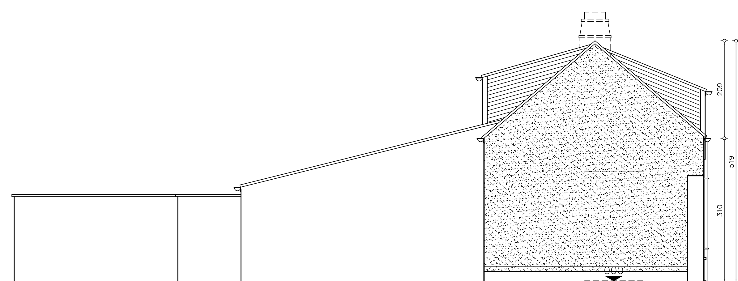
ZIJGEVEL LINKS SCHAAL 1/50
