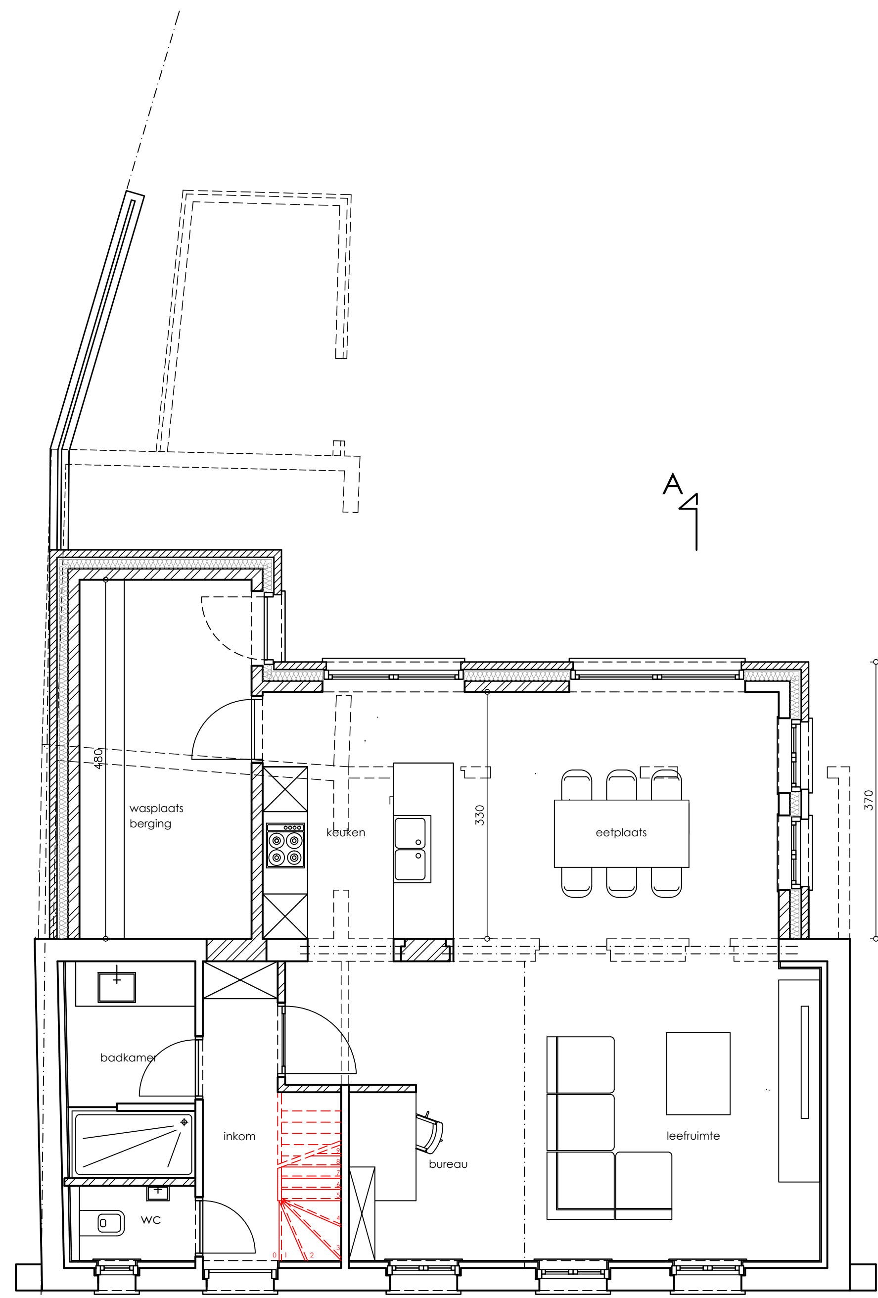
referentiepunt GRONDPLAN SCHAAL 1/50
