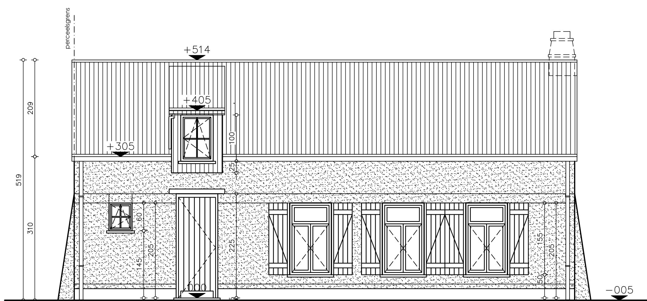
VOORGEVEL na verbouwing SCHAAL 1/50
