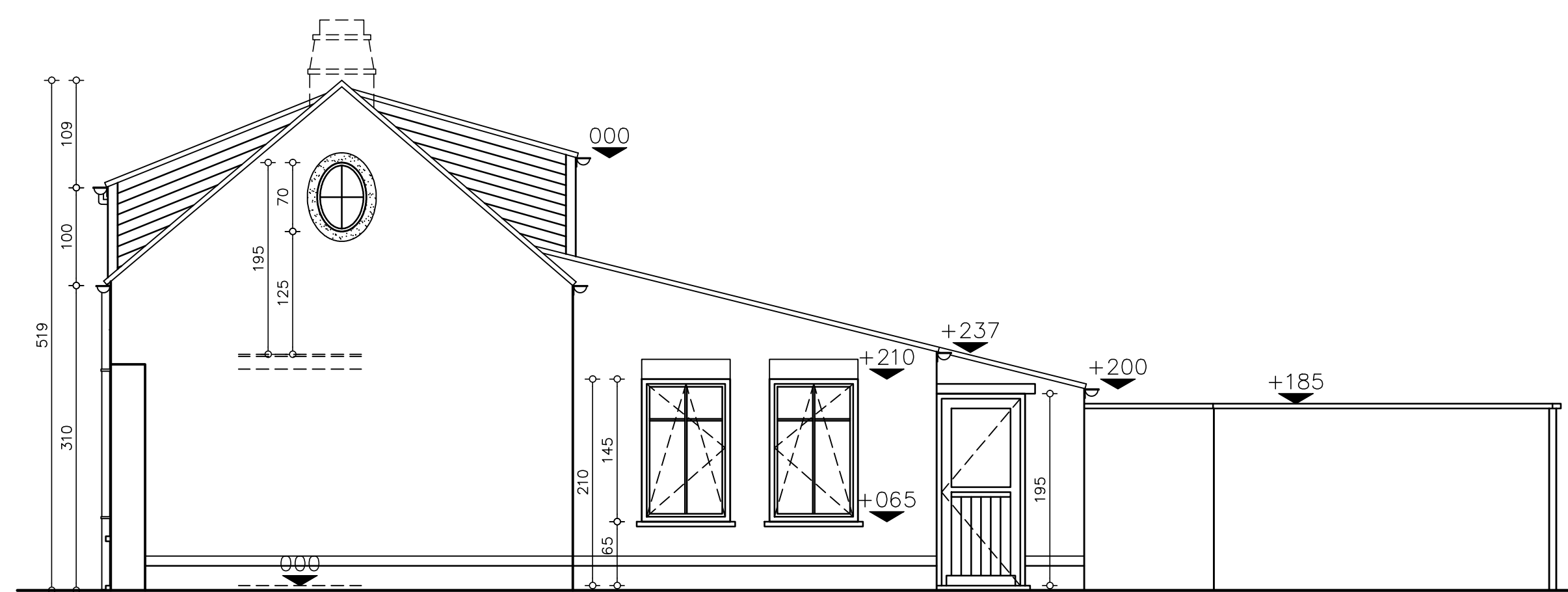
ZIJGEVEL RECHTS na verbouwing SCHAAL 1/50
