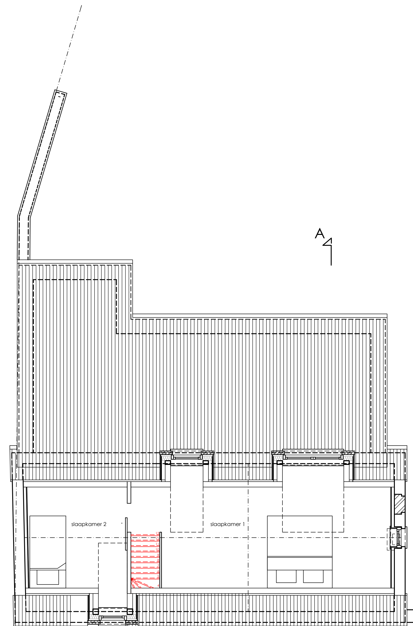
referentiepunt VERDIEPING SCHAAL 1/50
